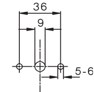
Bohrplan
