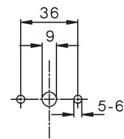
Bohrplan
