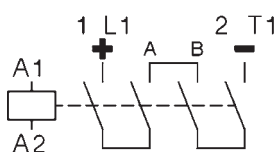
Schaltbild (4 Kontakte)
